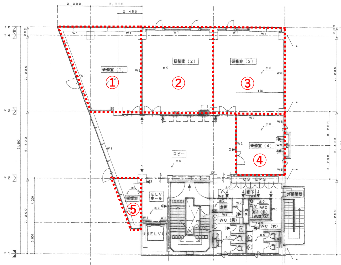
5階 平面図
